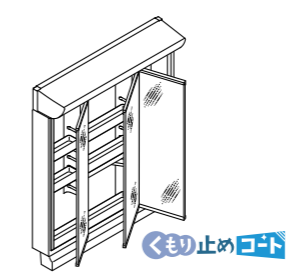
3面鏡(全収納・スタンダードLED) MVJ1-753TXSU
